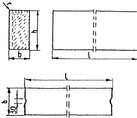
Tablica 1. Wymiary krawężników betonowych
