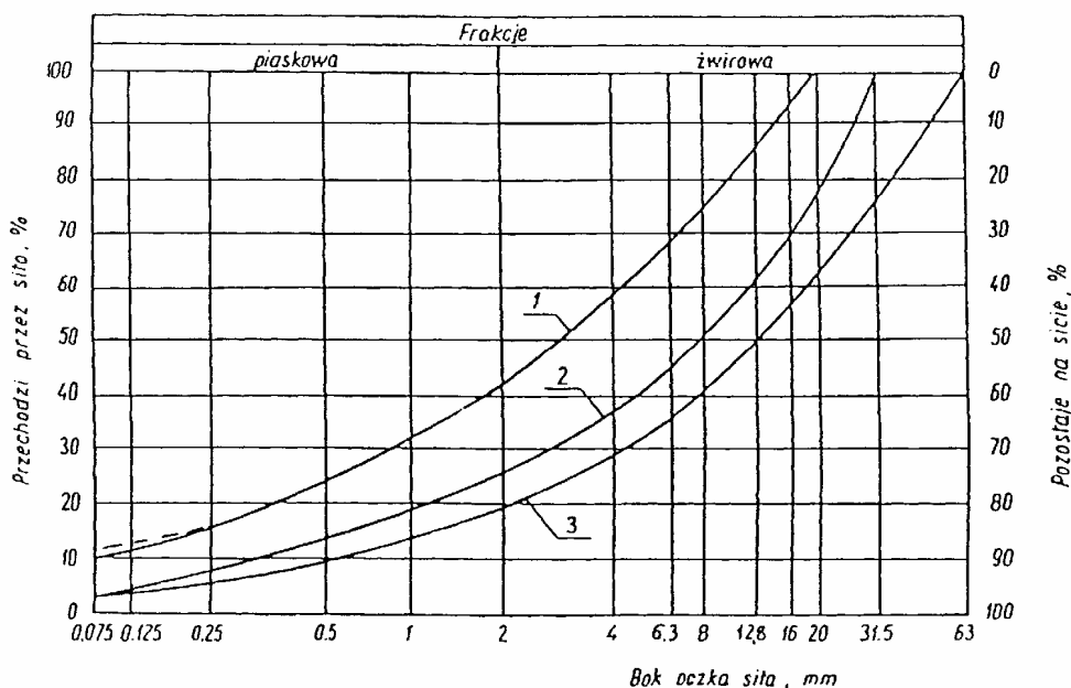
Rysunek 1. Pole dobrego uziarnienia kruszyw przeznaczonych na podbudowy wykonywane metodą stabilizacji mechanicznej 1-2 kruszywo na
