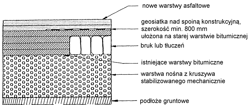
Rys. 3. Wzmocnienie nawierzchni asfaltowej w strefie poszerzenia nawierzchni
