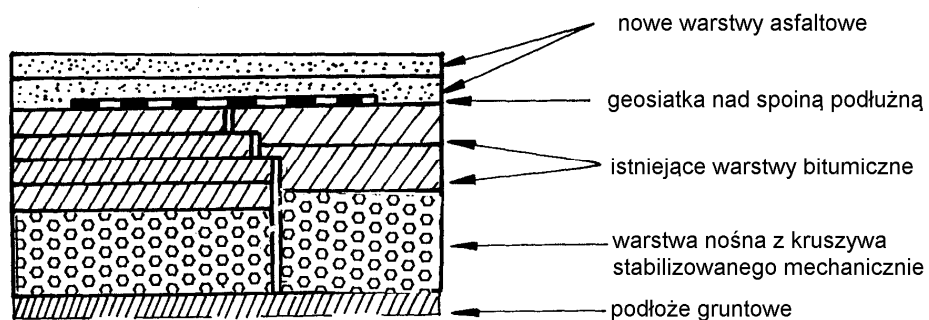
Rys. 3. Wzmocnienie nawierzchni asfaltowej w strefie poszerzenia nawierzchni
