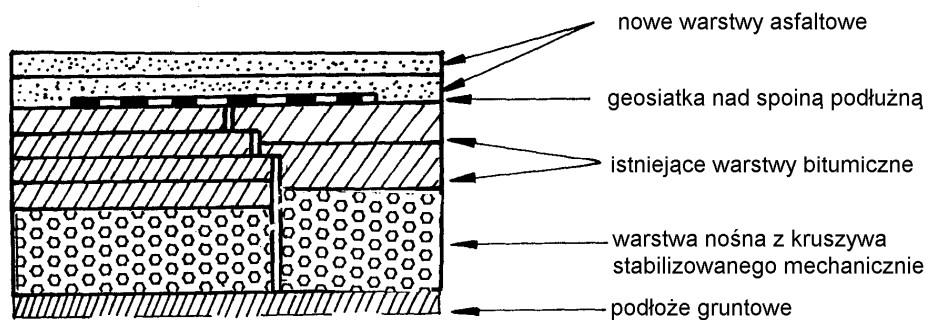
Rys. 3. Wzmocnienie nawierzchni asfaltowej w strefie poszerzenia nawierzchni a) wariant 1
